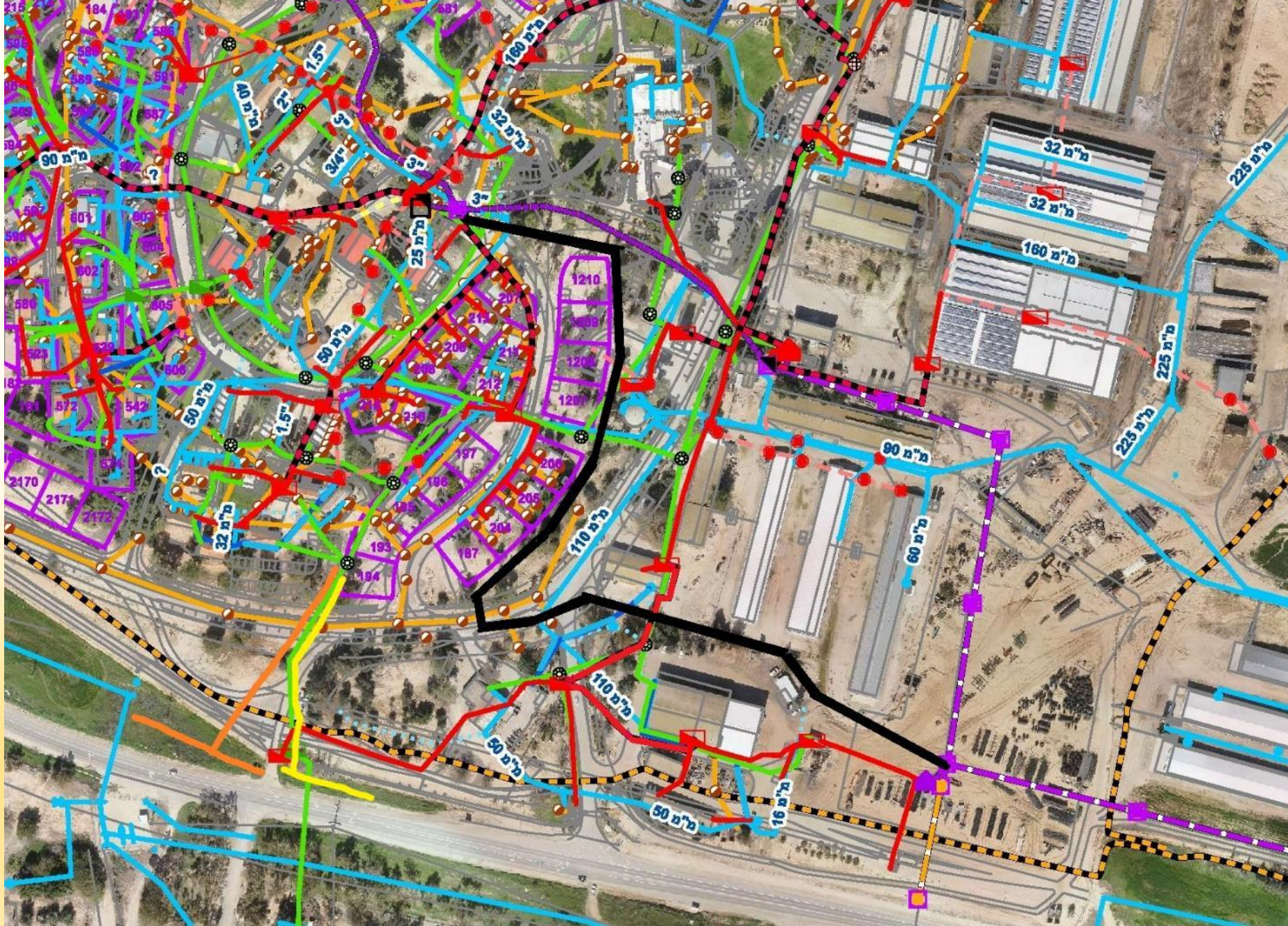
תוואי חפירה קו מתח גבוה עומק 1.8 מ' - שלב א'
